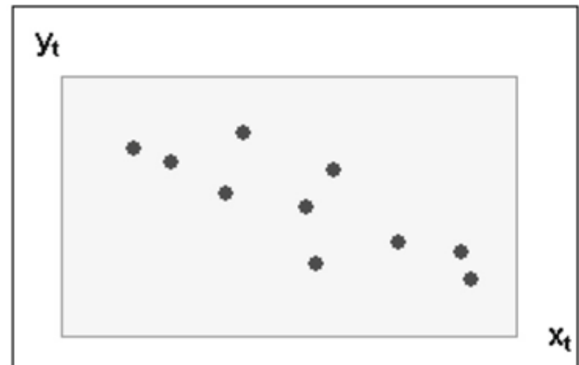
Streuungsdiagramm negativ korrelierter Beobachtungswerte
